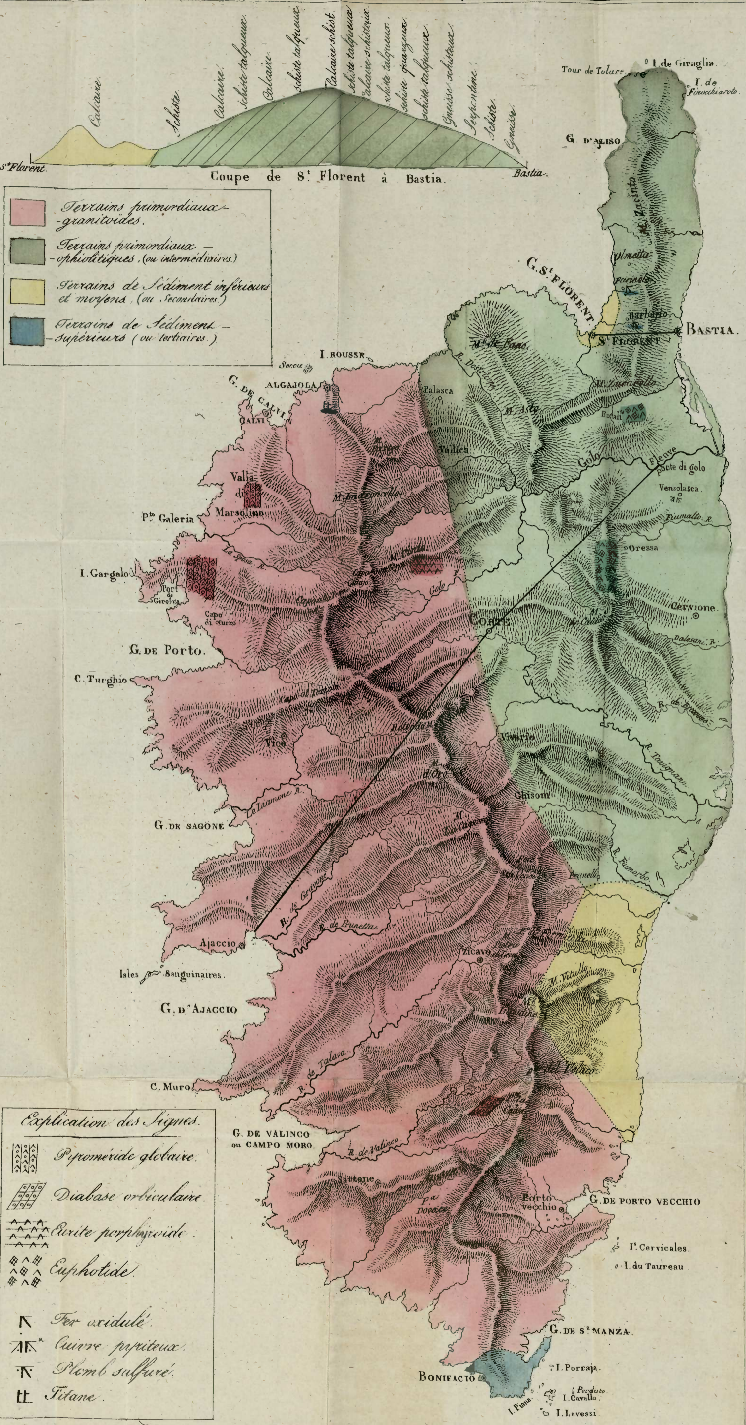
Essai d'une Carte géologique et Minéralogique de la Corse, par M. E. GUEYMARD, Ingénieur au Corps royal des Mines, 1820.
