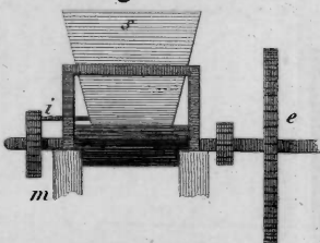
Projection verticale perpendiculaire à la fig. 1. des Cylindres cannelés et de la Tremie .
