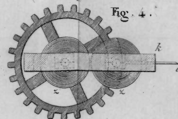
Projection Verticale sur une Echelle double d'une paire de Cylindres unis .
