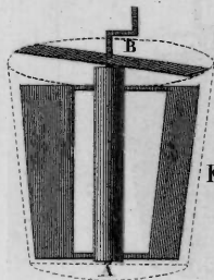
Tube à rincer (Dolly Tub) .
