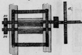
Projection horizontale d'une paire de Cylindres unis .
